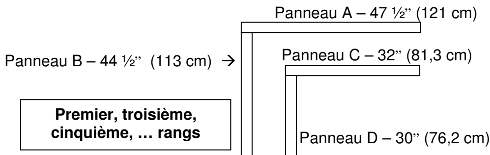
Fig. C-1. Assemblage des panneaux pour les rangs impairs
