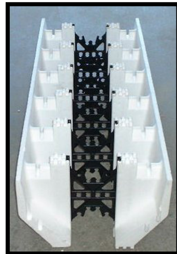
Fig. 14.2 On peut aussi doubler les panneaux d'appuis briques Integraspec® quand une surface de béton plus large est requise. Ceux-ci peuvent aussi être installés à différent niveau de l'un et de l'autre côté du mur IntegraSpec .
