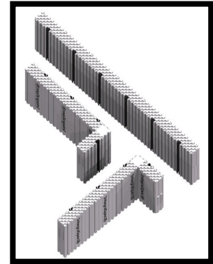
Fig. 9.1 Disposition du mur en T (panneaux de coins intérieurs à 90° et panneaux standard)
