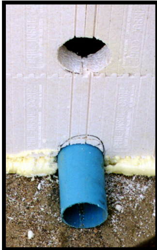
Fig. 12.1 Tuyau installé à l'endroit approprié. L'ouverture pour les services est centrée entre les inserts (plaques d'identification sur les panneaux IntegraSpec® en laissant un écart d'au moins 1" (2,5 cm) pour les barres d'armature.
