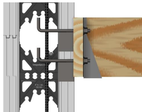
Fig. 17.5 Boulons d'ancrage pour fixer la lisse de plancher, le balcon, terrasse et l'avant-toit
