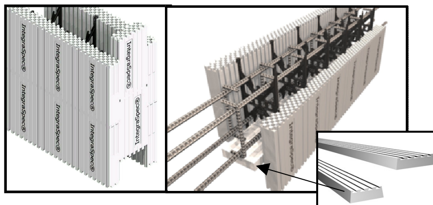
Fig. 10.5 IntegraBuck (à gauche); IntegraHeader (bas à droite) (des panneaux standards coupés peuvent aussi être utilisés comme substitue d'IntegraBuck et ou IntegraHeaders)
