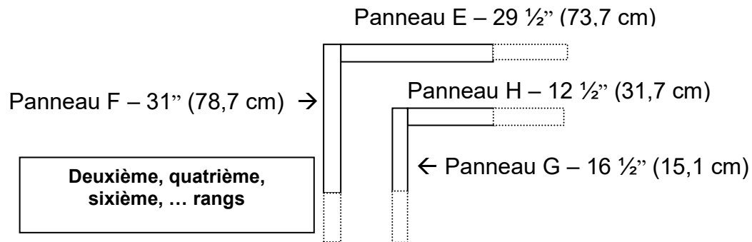
Fig. C-3. Assemblage des panneaux pour les rangs pairs
